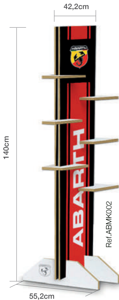
Totem display 6 posições
