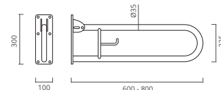
BARRA DE APOIO Ø35MM REBATÍVEL C/ PORTA ROLOS
