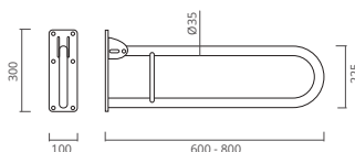
BARRA DE APOIO Ø35MM REBATÍVEL
