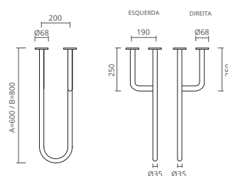
BARRA DE APOIO Ø35MM 3 APOIOS
