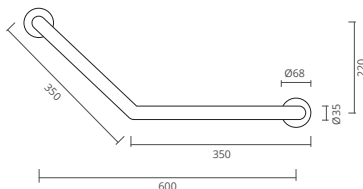
BARRA DE APOIO Ø35MM 135°
