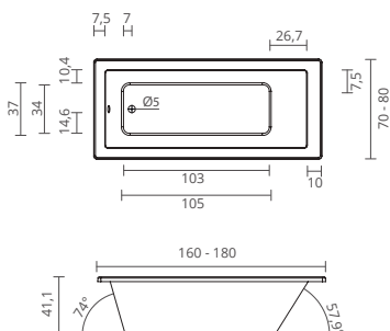
BANHEIRA ACRÍLICA RECTANGULAR COMPLEMENTAR COM PAINÉIS FRONTAIS E LATERAIS (VER PÁGINA 242)
