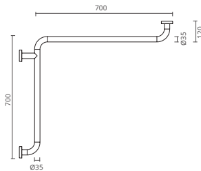
BARRA DE APOIO Ø35MM 90°
