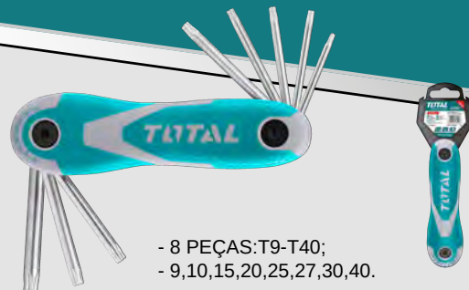
JOGO CHAVE SEXTAVADA TROX. PROF. THT1061846
