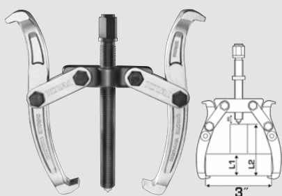
SACA ROLAMENTOS 2 PERNAS
