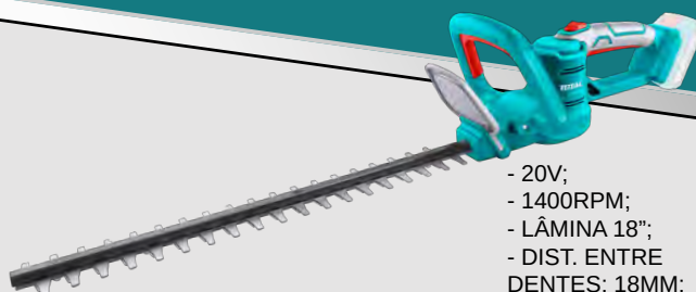
CORTA SEBES THTLI2001
